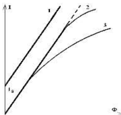
Рис.2. Световая характеристика фотодиода.
