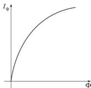
Рис.1. Световая характеристика фоторезистора.
