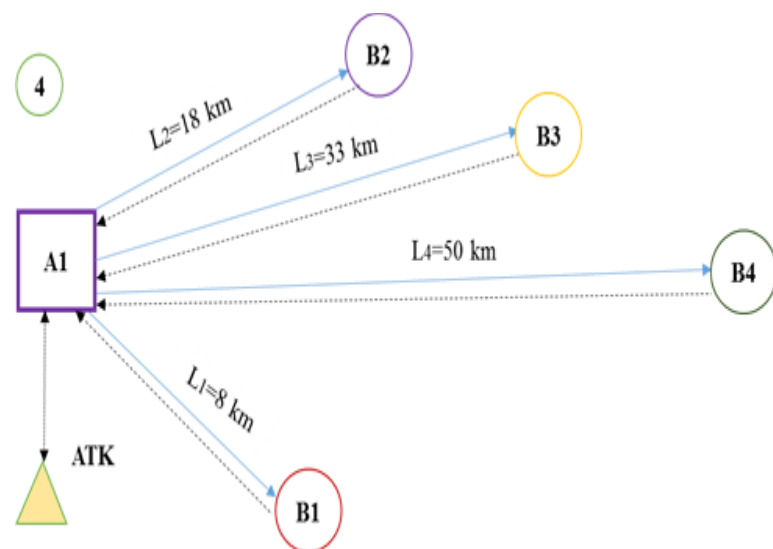
1-rasm. Yuk jo'natuvchi va qabul qiluvchilarning joylashish sxemasi
