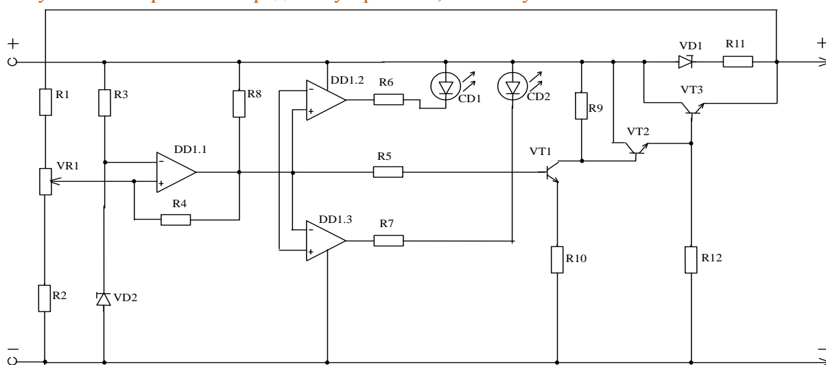
Рисунок 2 Принципиальная схема контроллера, заряжающего аккумулятор от солнечной батареи и поддерживающего ее на уровне 13 вольт. R1,R2-33K; R3-510; R4-1M; R5-1K; R6,R7-470; R8-1K; R9-1,2K; R10-120; R11-100; R12-300; VD1,VD2-KC162; DD1-LM339; VR1-50K; VT1-KT315; VT2-KT605; VT3-KT819.
