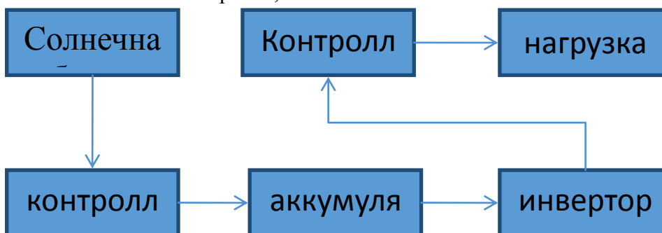
Рисунок 3. Идеальная блок-схема для энергоснабжения потребителя солнца
