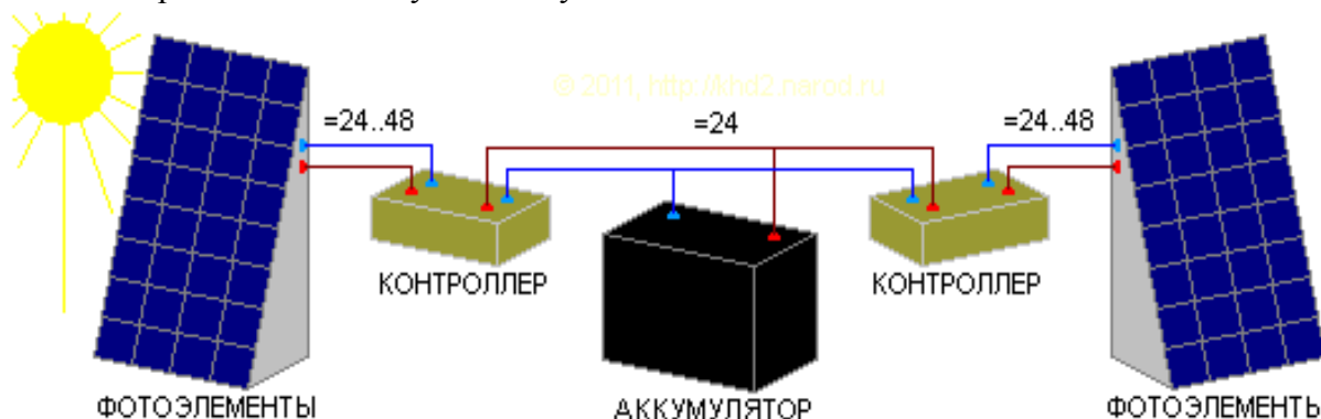
Рисунок 1 Изображение зарядного устройства, используемого в солнечной панели.
